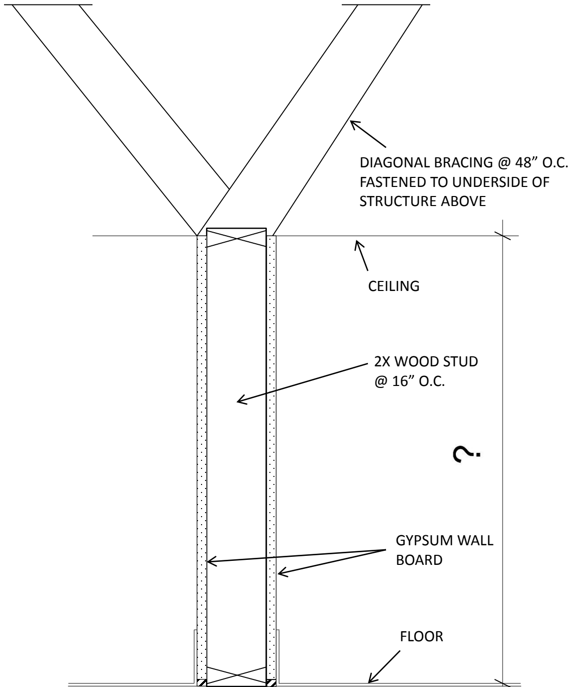
WOOD STUD PARTITION
