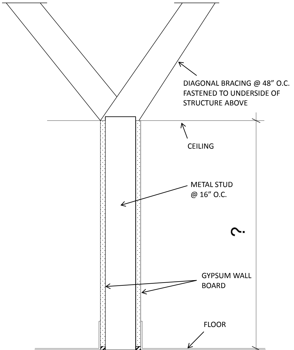
METAL STUD PARTITION
